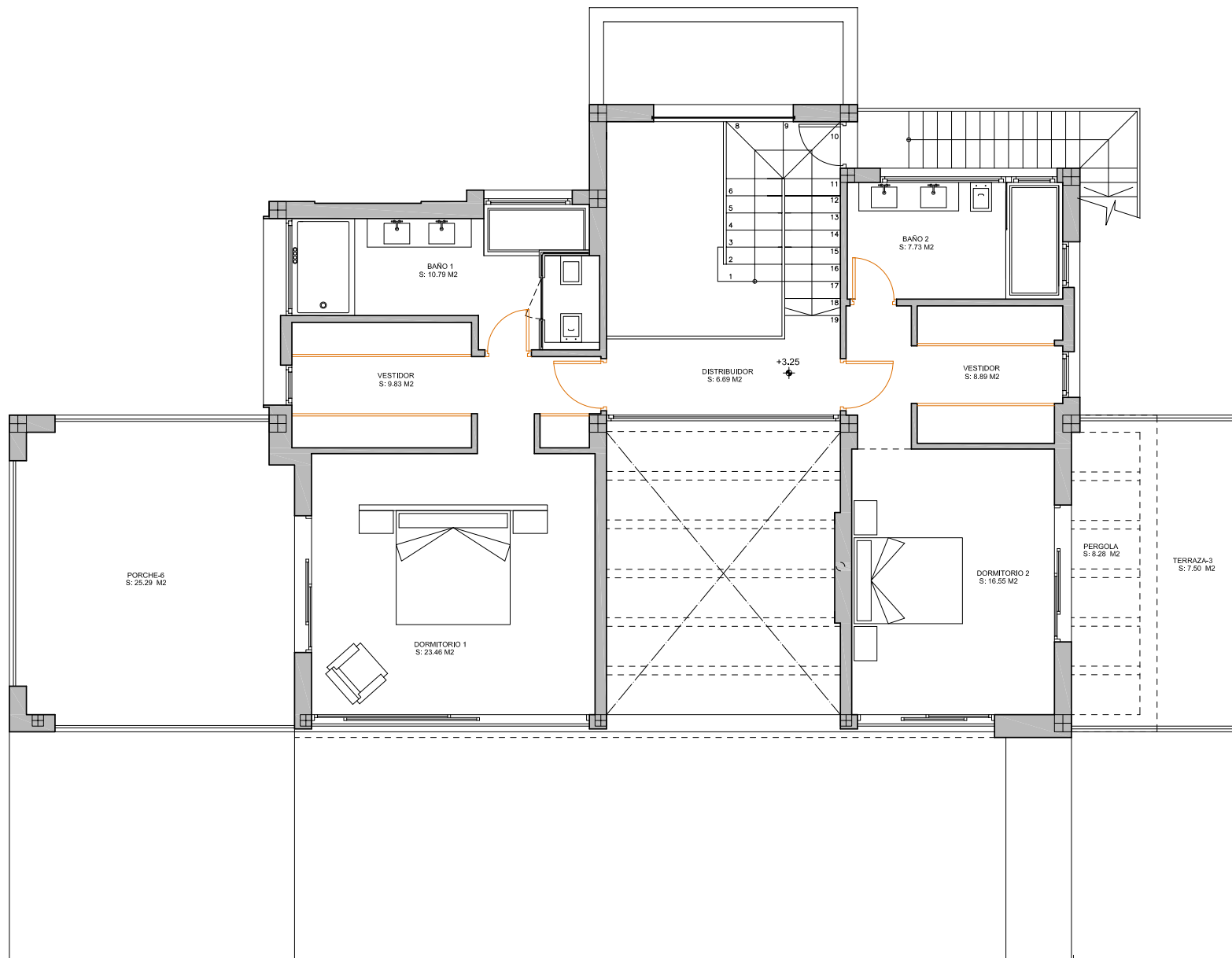
FIRST FLOOR PRIMERA PLANTA
